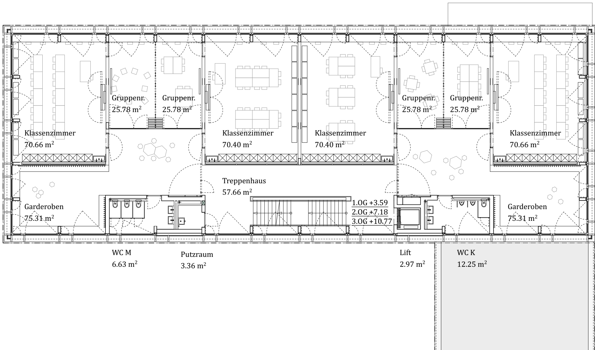
SCHULHAUS 4 Grundriss 1. - 3. Obergeschoss
