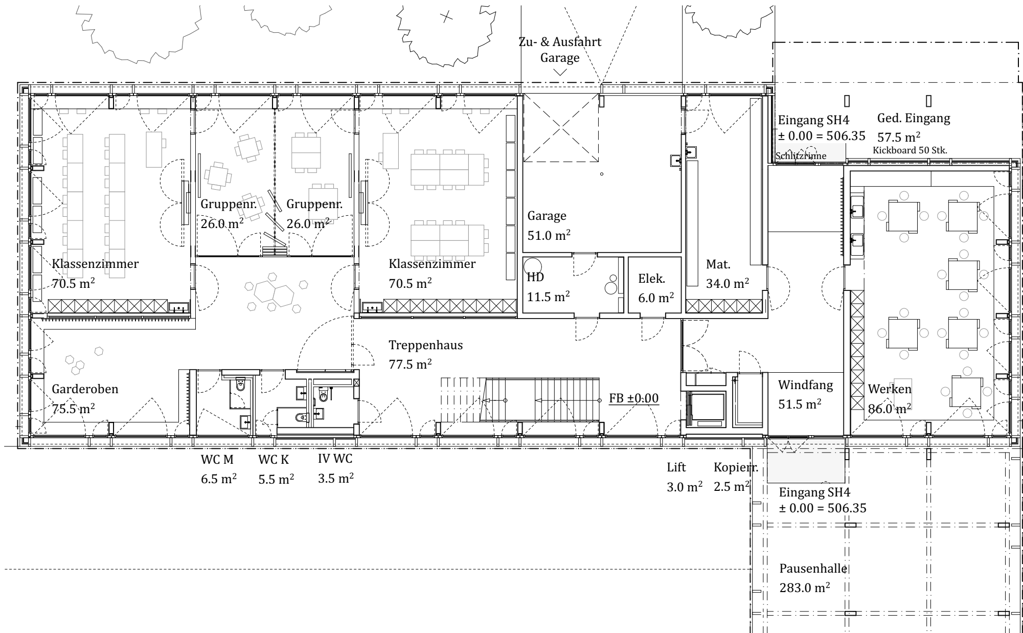
SCHULHAUS 4 Grundriss Erdgeschoss
