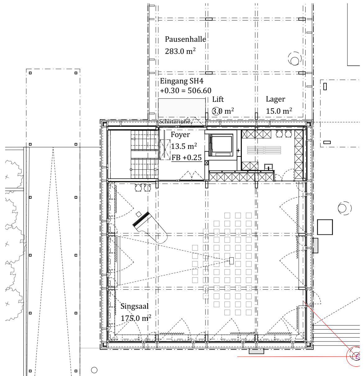
Grundriss Erdgeschoss
